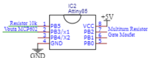
Gambar 6. Rangkaian ATtiny85
