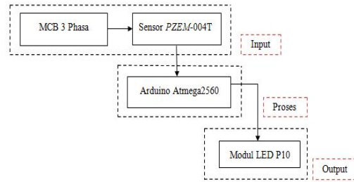
Gambar 5. Diagram blok sistem perangkat keras
