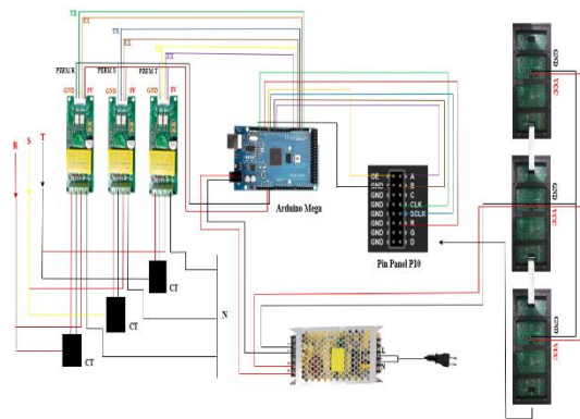
Gambar 6. Skematik rangkaian
